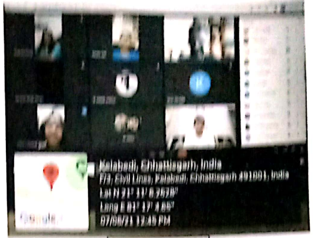
participants
