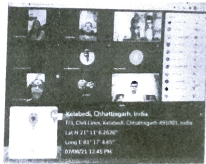
participants
