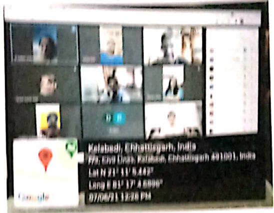
participants
